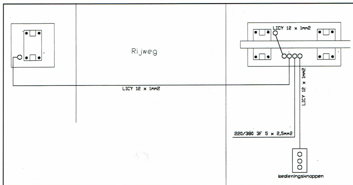
Kabelschema
