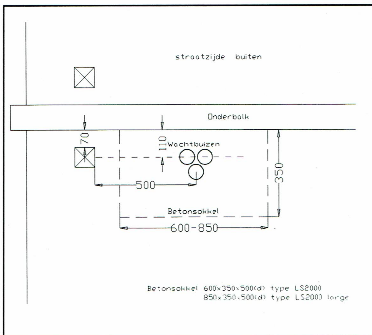
Betonschema
