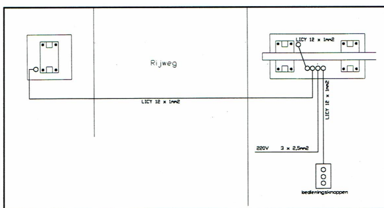
Kabelschema
